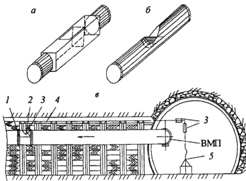
Рис. 1. Устройство для разгаживания тупиковых горных выработок: а, б - схемы устройства; в - схема установки; 1 - патрубок;
