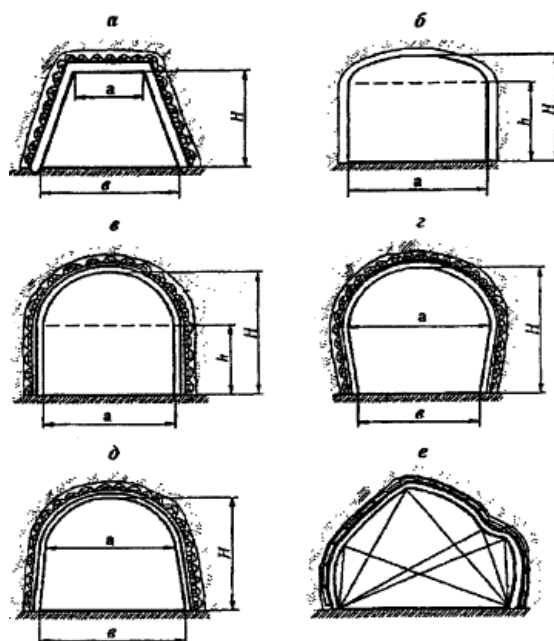
Рис.2. Поперечные сечения горных выработок: а - трапециевидное сечение; б - коробковый свод; в - при полуциркулярном
